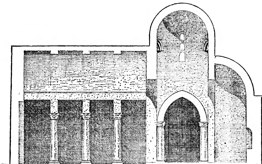
L'église du Deir-el-Malak . — Coupe longitudinale. — Restauration.
