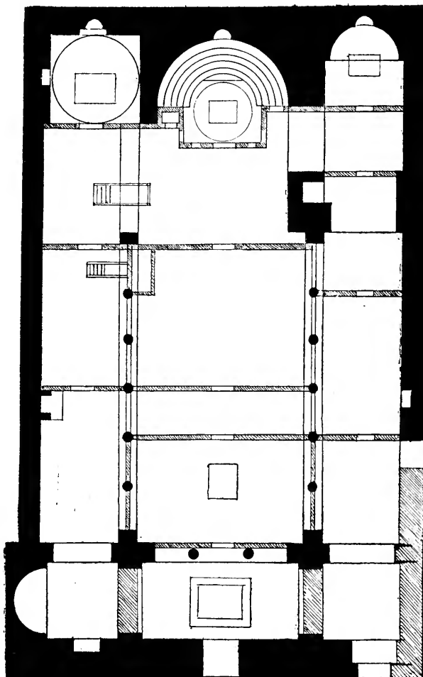
L'église du Deir-Abou-Sergah . — Plan.
