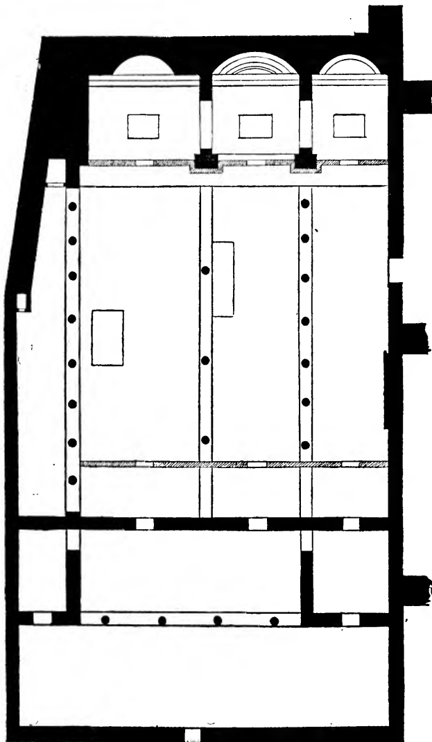
L'église du Mohallakah. — Plan.
