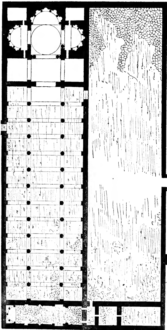
L'église du Deir-el-Abiad . — Plan restauré.
