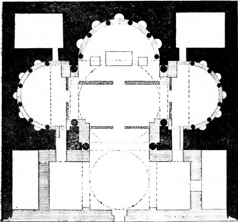
L'église du Deir-el-Abiad . — Plan du sanctuaire.
