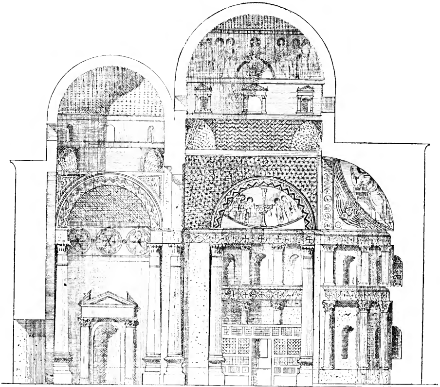
L'église du Deir-el-Abiad . — Coupe longitudinale. — Restauration.
