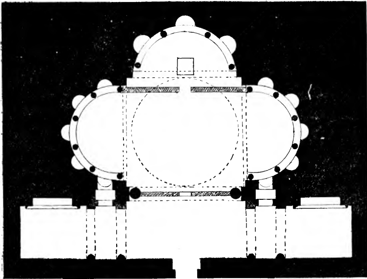
L'église du Deïr-el-Akhmar . — Plan du sanctuaire.
