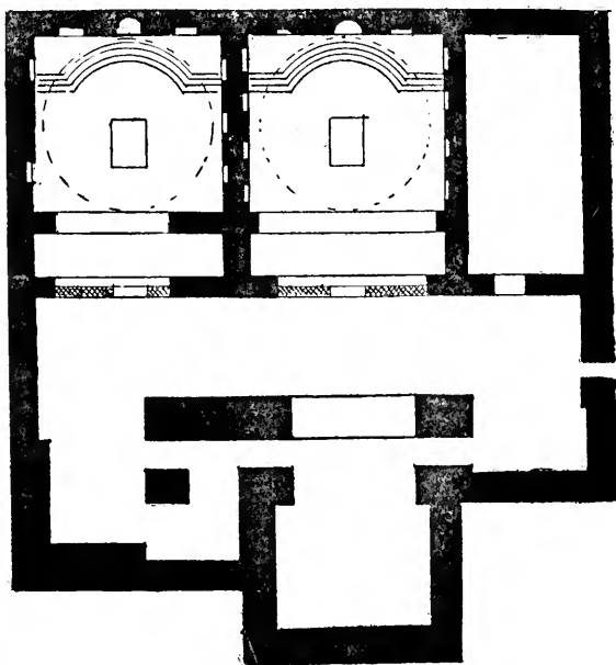
L'église du Deir-abou-Makur . — Plan.
