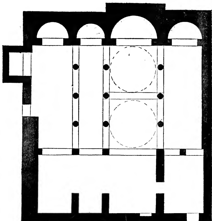
L'église du Deir-el-Azam . — Plan.
