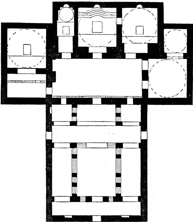
L'église de l'Amba-Beschaï. — Plan.
