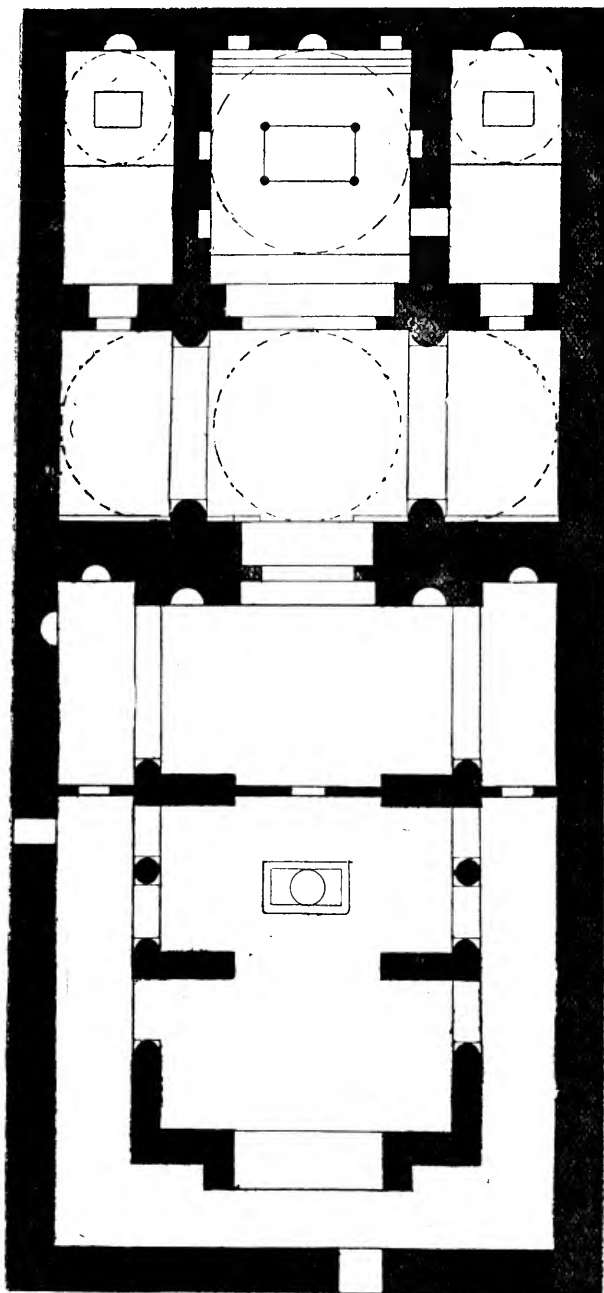
L'église du Deir-es-Souriani . — Plan.
